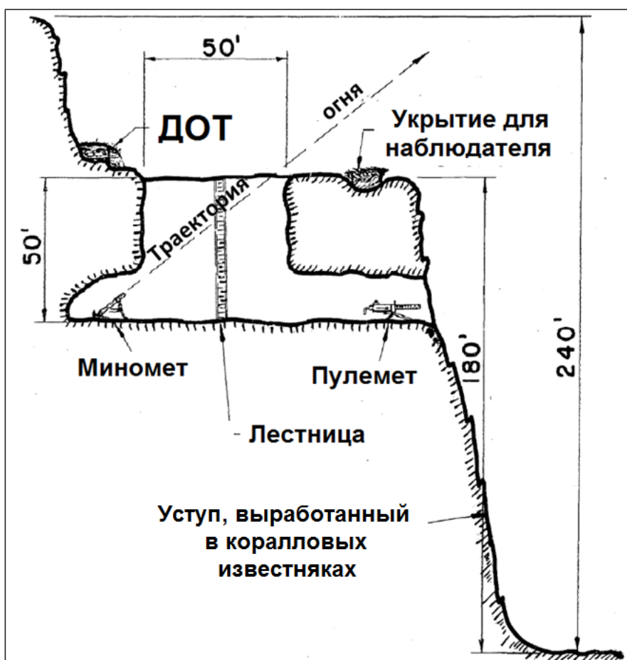
Схематический разрез через скрытый в пещере пункт обороны японцев. Размеры указаны в футах
